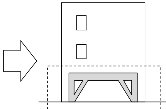
1階のピロティ階の耐震補強
