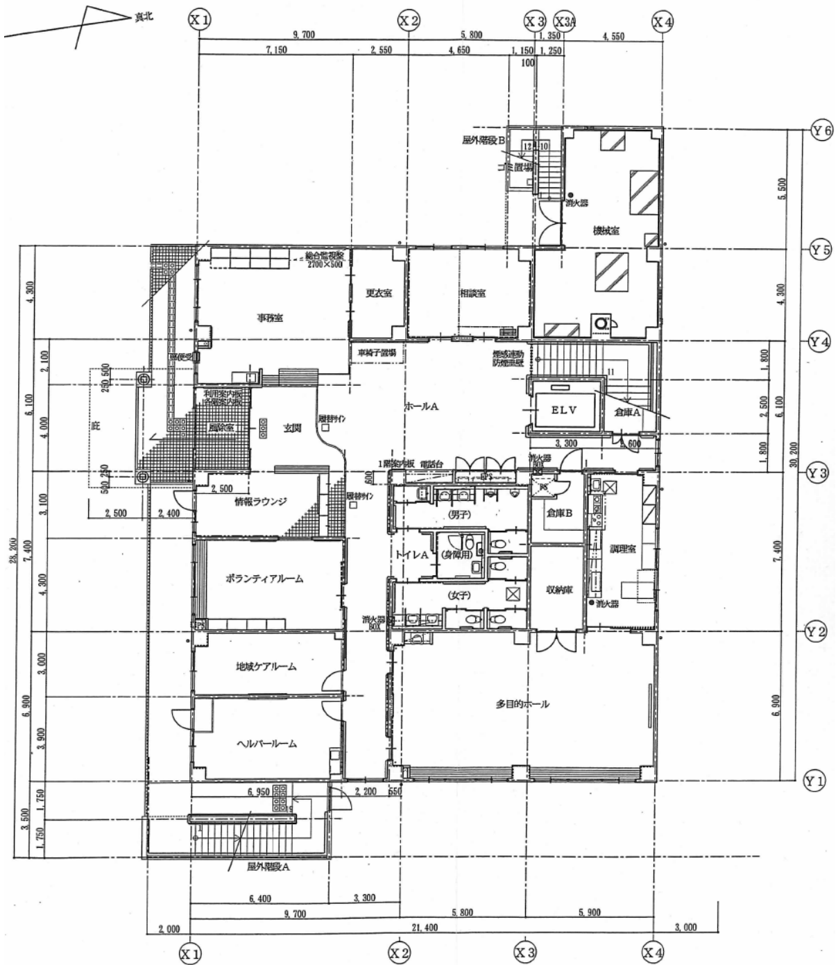
1階平面図
