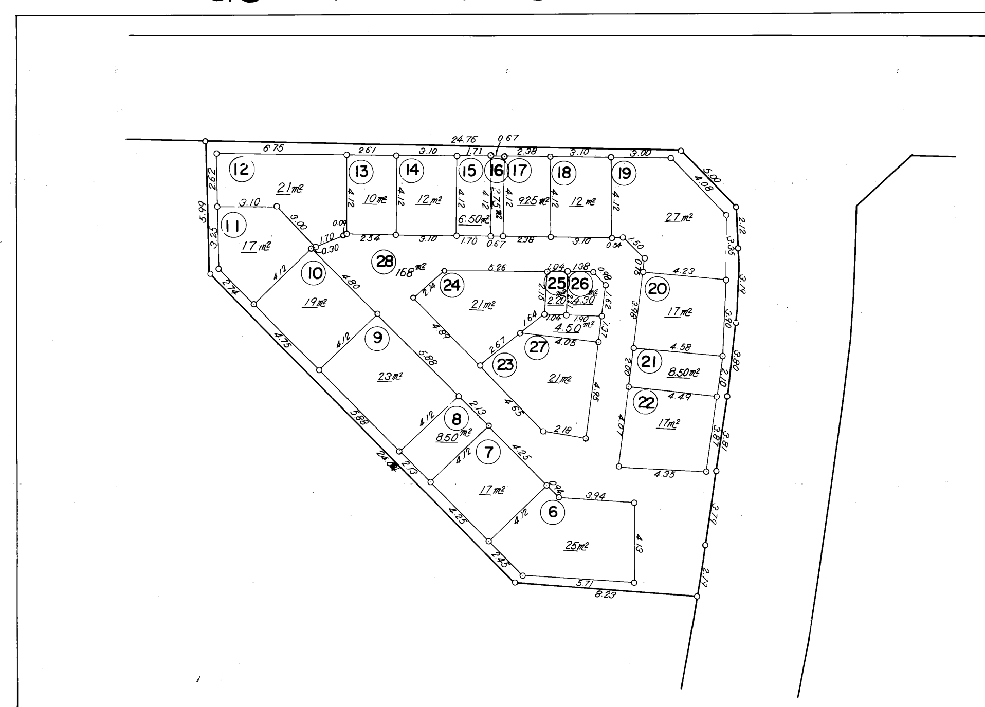
集合墓地確定図 S=1:200
