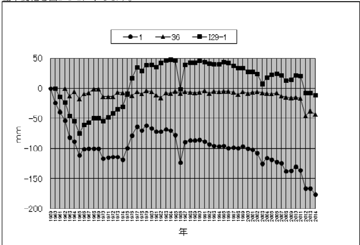
図 2-1-2 鶴見区水準点経年変化
