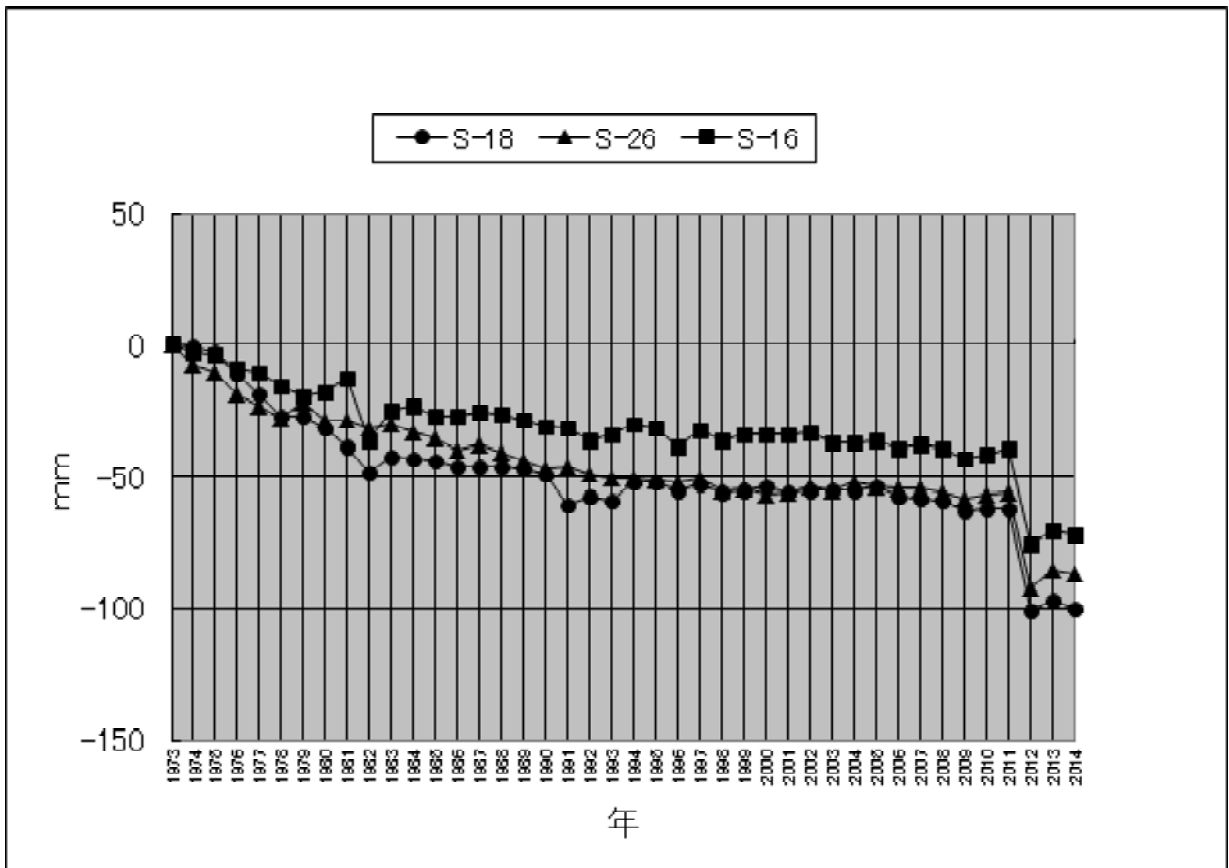
图 2-1-19 瀬谷区水准点经年变化
