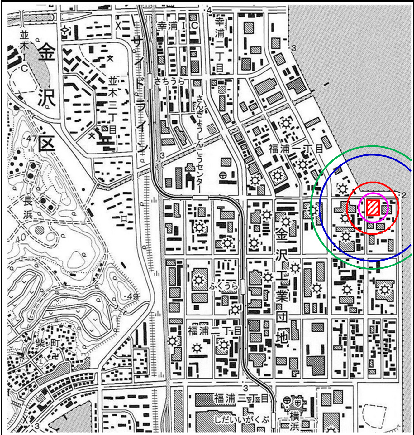
図-6(2) 予測条件別大気質最大着地濃度出現位置(一時間値) 二酸化窒素以外の項目
