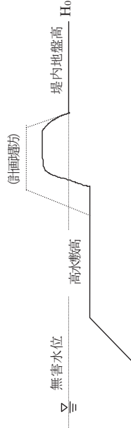
図-2.4 無害流量設定における未改修時点の堤防の評価方法
