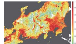
宇宙から見た日本の夏(2018年8月1日) ©JAXA/EORC
