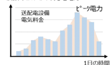
複数のEVバスの充電方法
