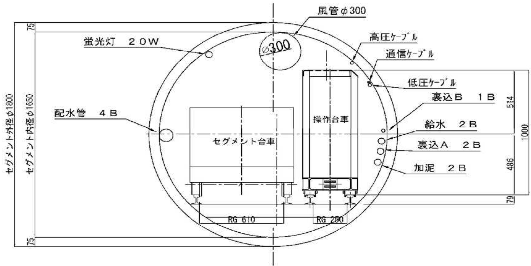
一次覆工時の坑内断面図（参考図）
