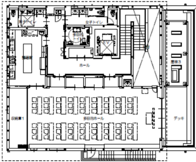
2階平面図 1/100
